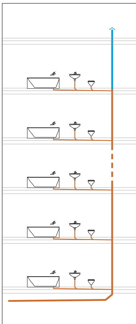
Ensiötuuletettu järjestelmä
