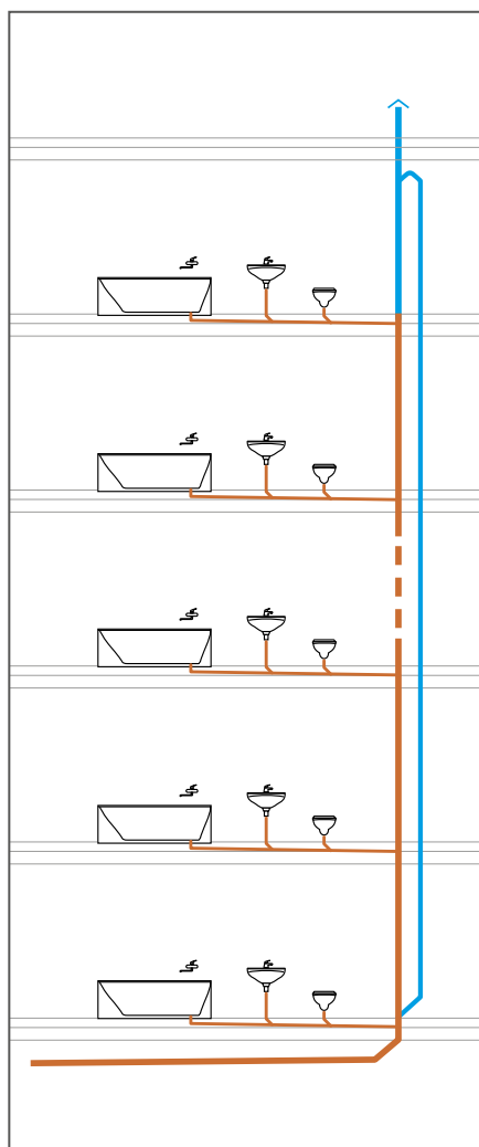
Rinnakkaistuuletettu järjestelmä
